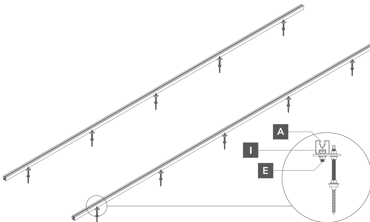
Rys. 6. Mocowanie szyny montażowej do adaptera montażowego
