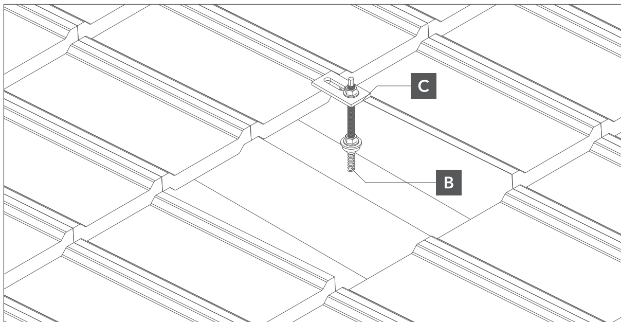
Rys. 4. Mocowanie śruby z gwintem podwójnym do krokwi
